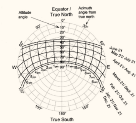
Sun Path Diagram, 32° S Latitude Source: Harvesting Rainwater
